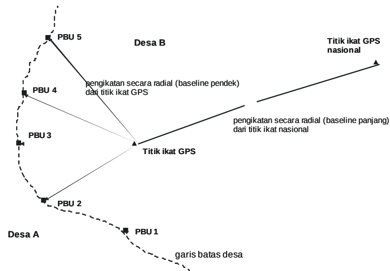
Gambar 15. Pembuatan Titik Referensi Baru
