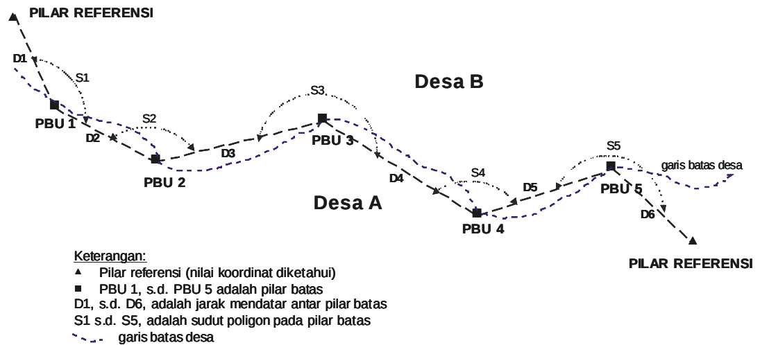
Gambar 14. Poligon Terbuka
