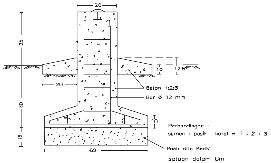
(a) Konstruksi Pilar
