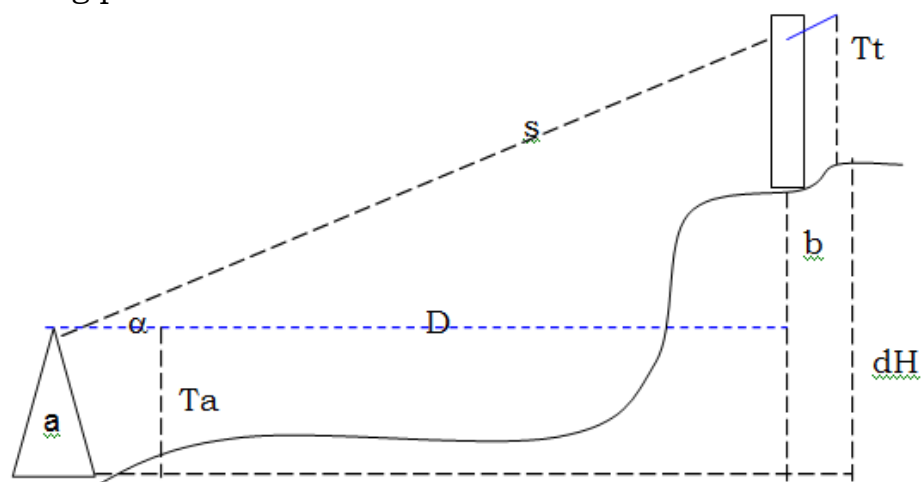
Gambar 17. Pengukuran Tachimetri
